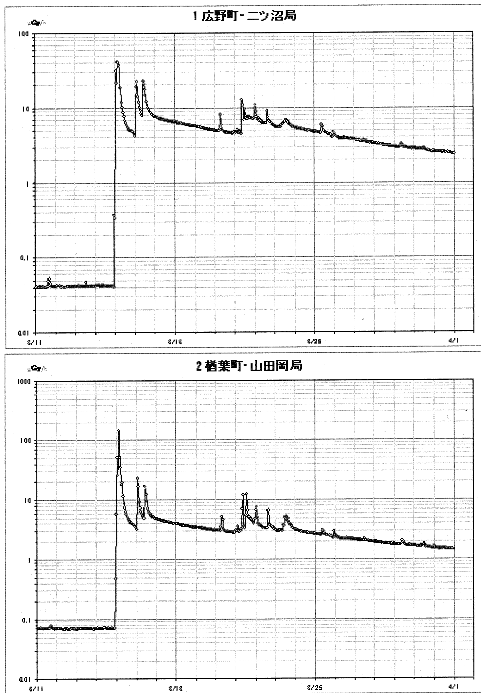
図 C1-4 (7/9) 福島県モニタリングポストの線量率
