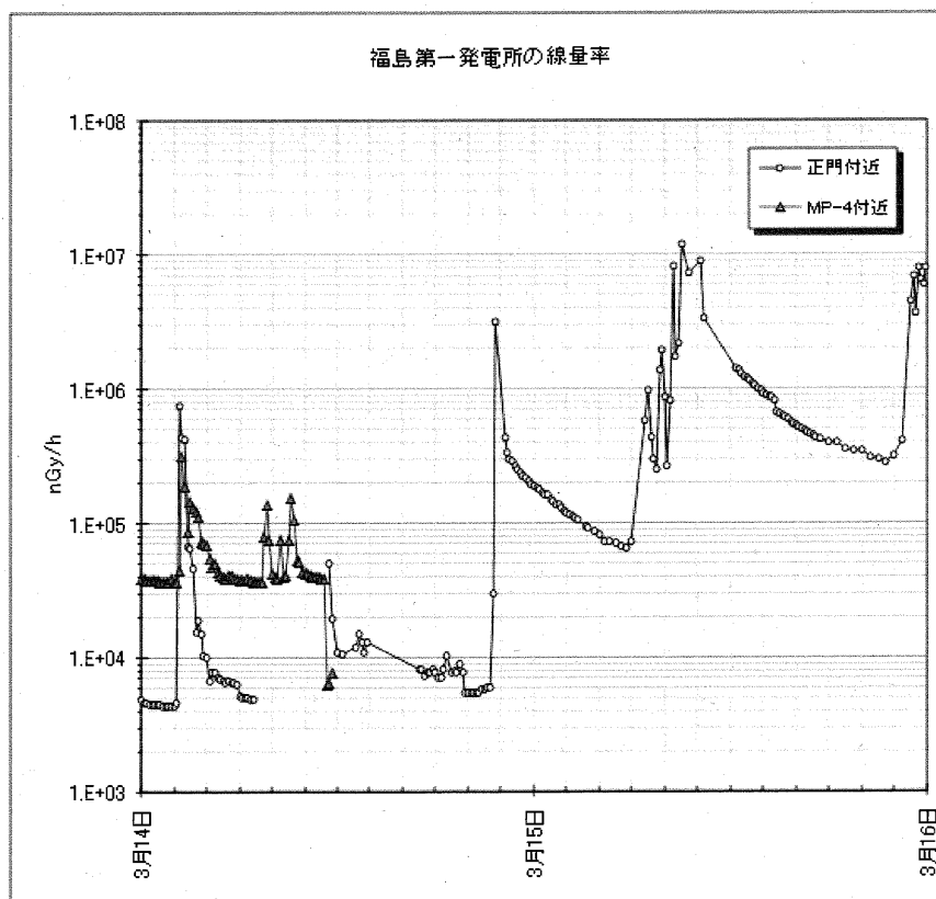
図 C1-1 (2/7) 福島第一発電所構内の線量率 (3月14日—15日)
