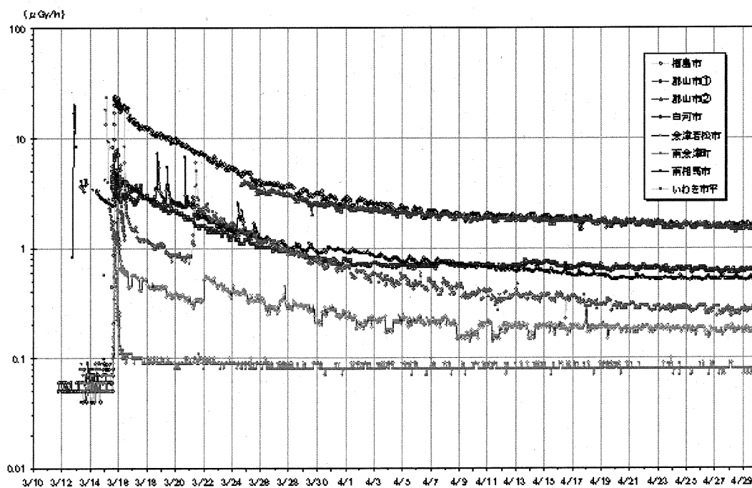
図 C1-6 福島県・県内7方部環境放射能測定結果
