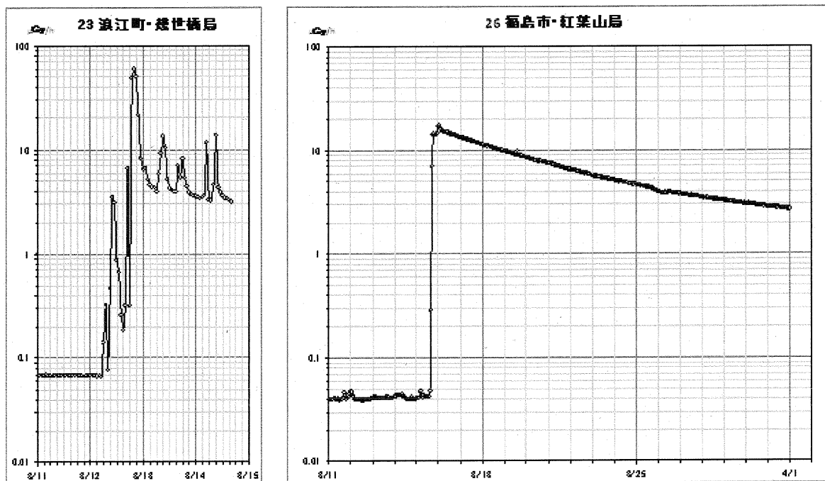
図 C1-4 (6/9) 福島県モニタリングポストの線量率
