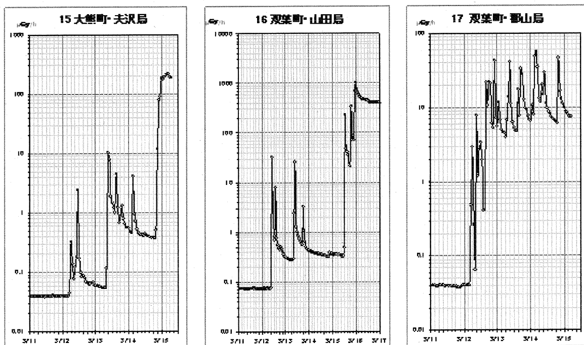
図 C1-4 (4/9) 福島県モニタリングポストの線量率
