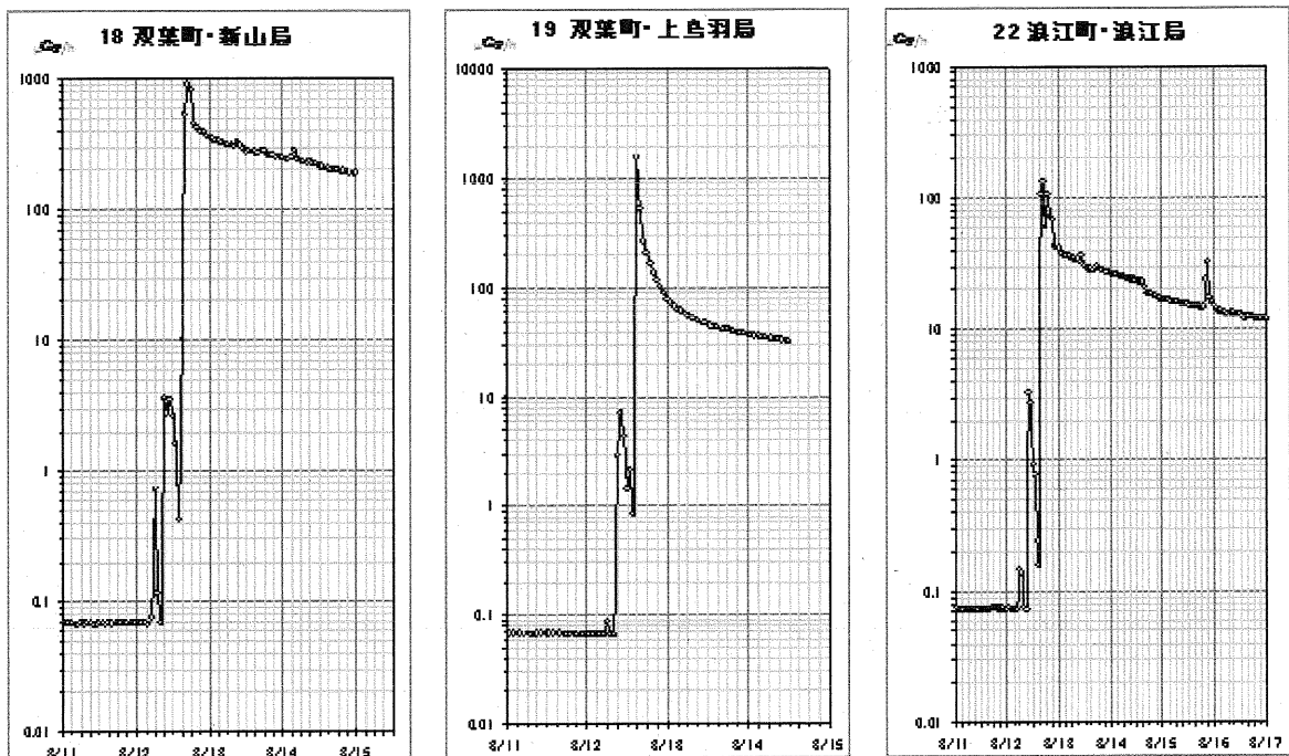
図 C1-4 (5/9) 福島県モニタリングポストの線量率
