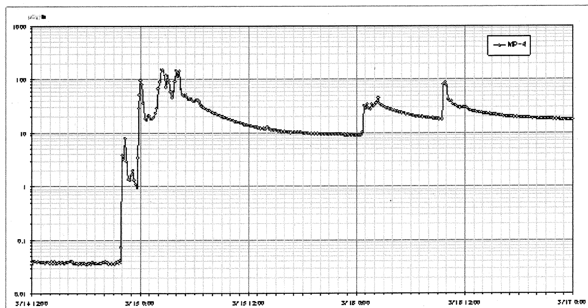
図 C1-2 (2/2) 福島第二発電所における線量率（平成 23 年 3 月 14 日～16 日）
