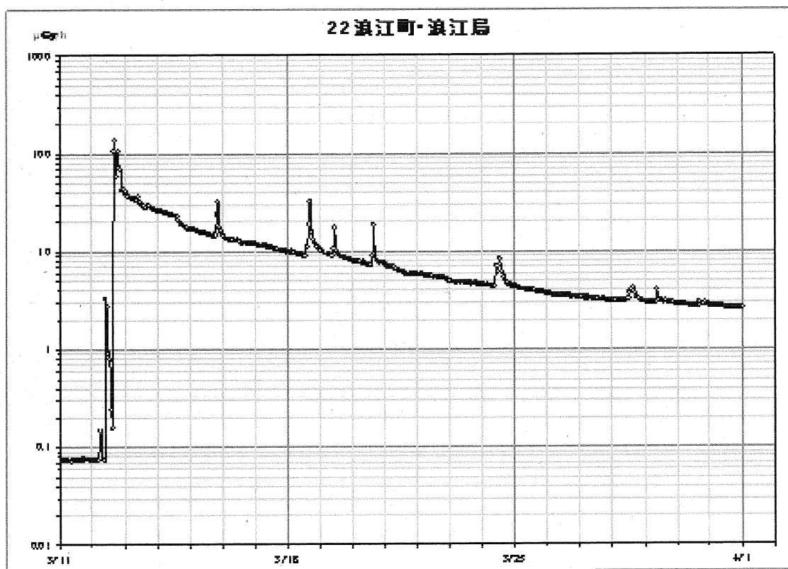
図 C1-4 (9/9) 福島県モニタリングポストの線量率
