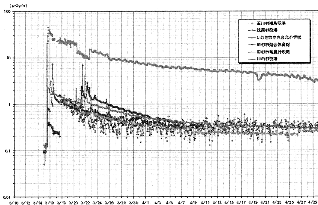
図 C1-5 福島県・20 km～50 km圏付近環境放射能測定結果
