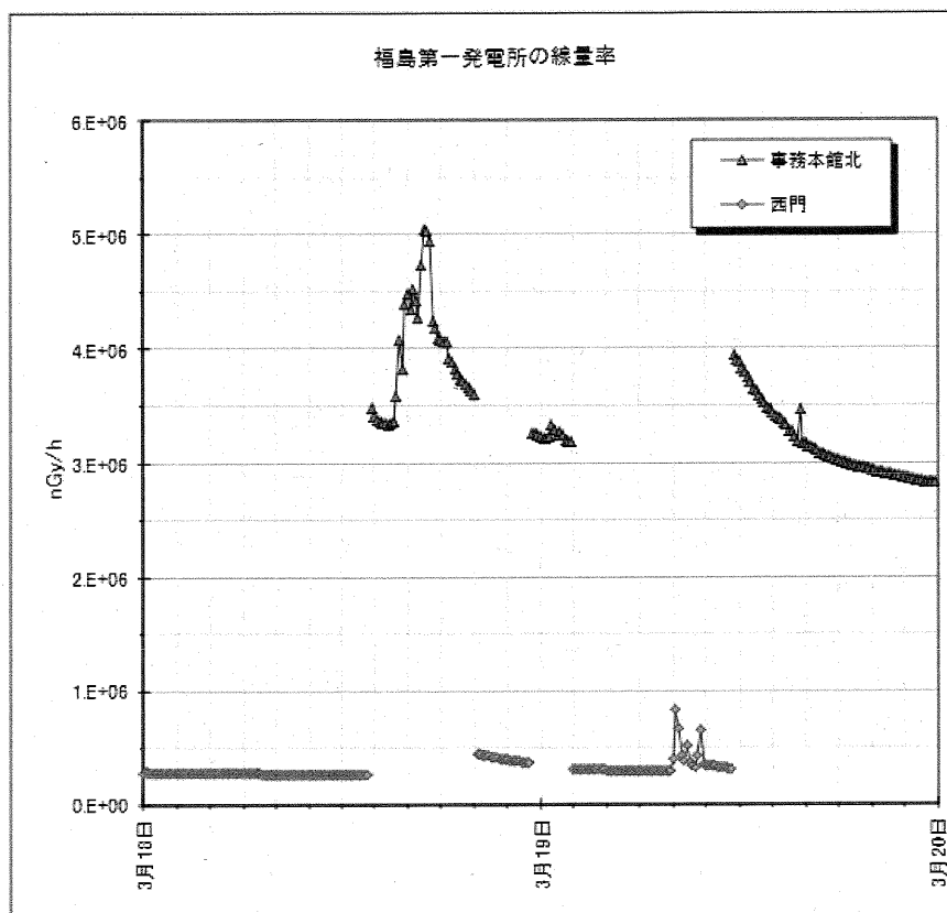
図 C1-1 (4/7) 福島第一発電所構内の線量率 (3月18日—19日)
