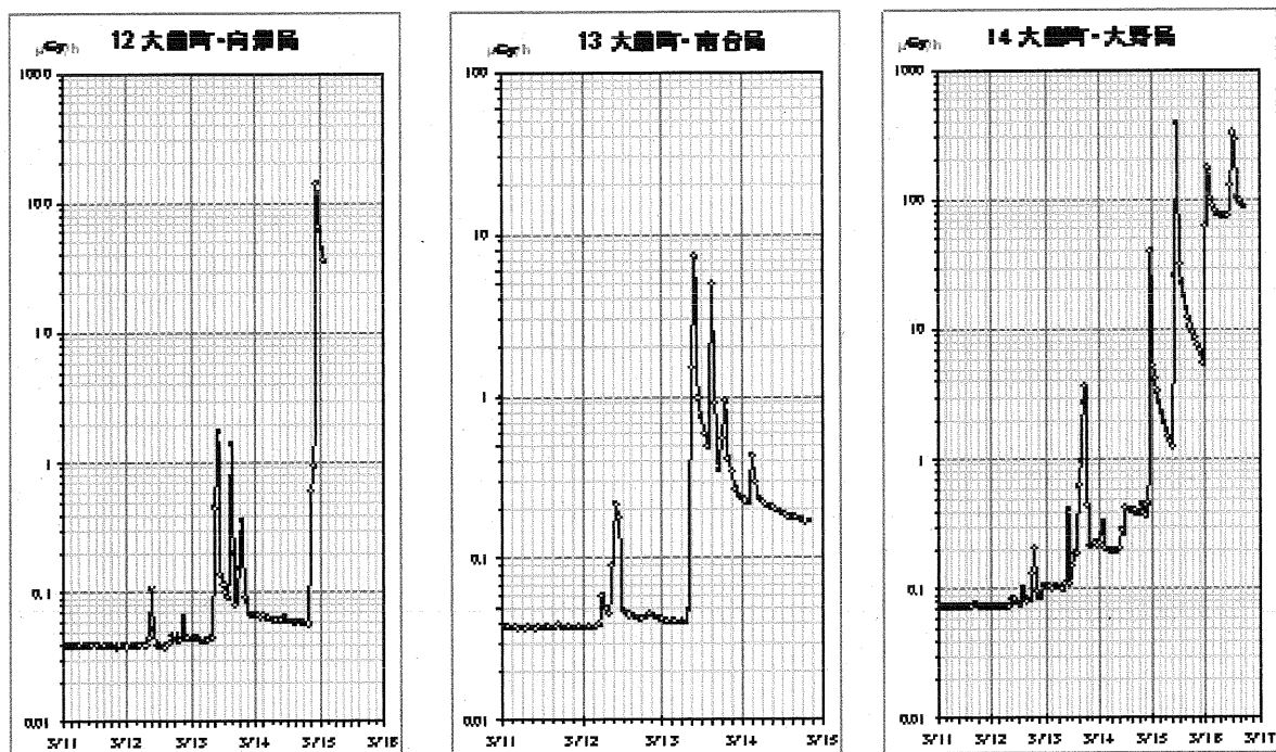
図 C1-4 (3/9) 福島県モニタリングポストの線量率
