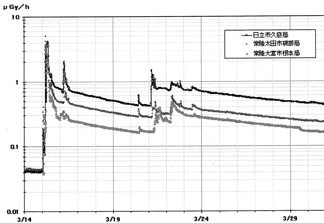
図 C1-7 茨城県のモニタリングポストの線量率
