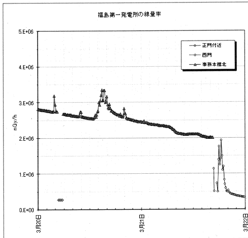
図 C1-1 (5/7) 福島第一発電所構内の線量率 (3月20日～21日)
