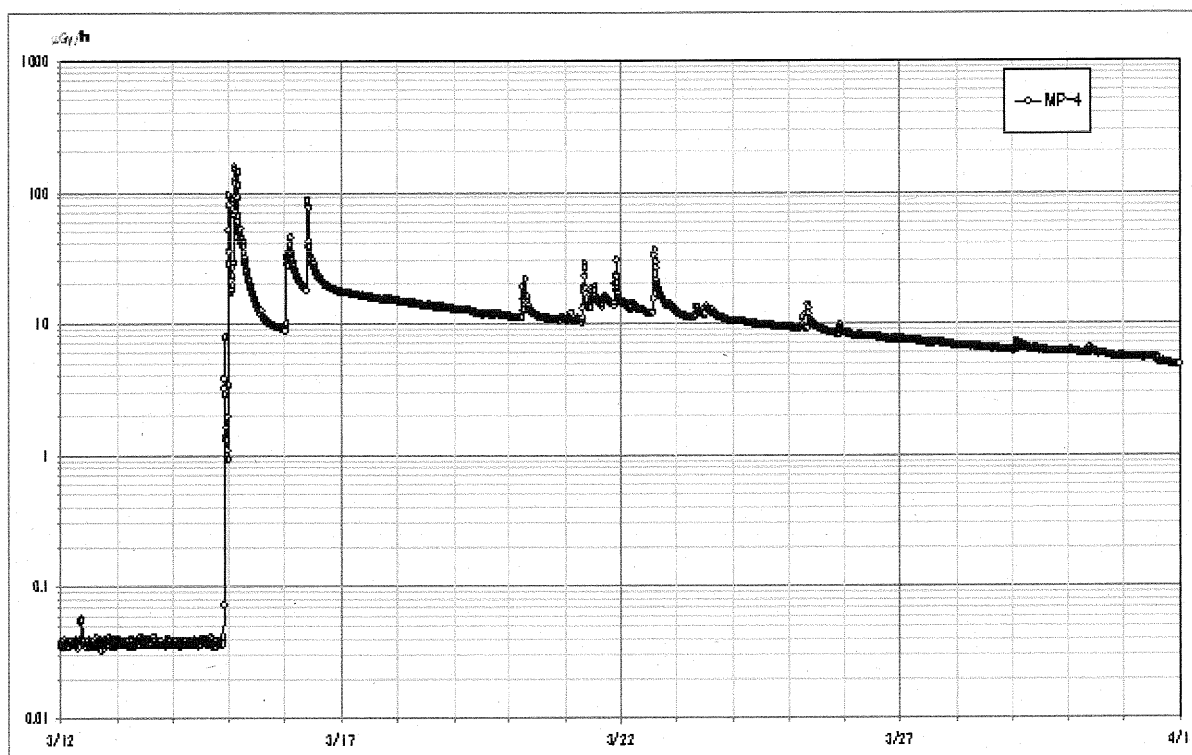
図 C1-2 (1/2) 福島第二発電所における線量率（平成 23 年 3 月 12 日～31 日）
