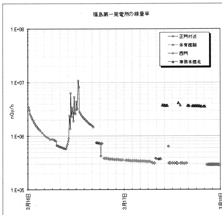
図 C1-1 (3/7) 福島第一発電所構内の線量率 (3月16日—17日)
