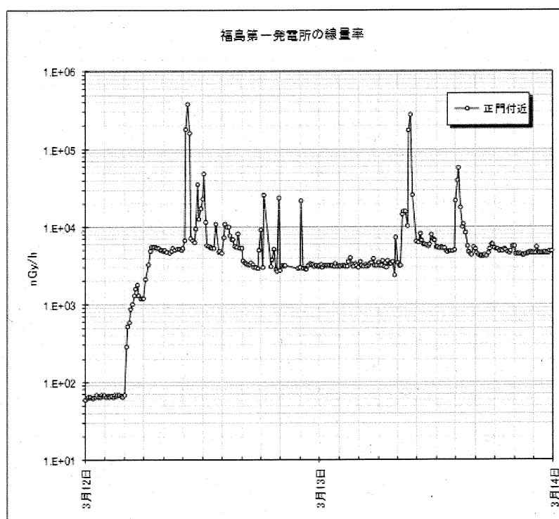
図 C1-1 (1/7) 福島第一発電所構内の線量率 (3月12日—13日)
