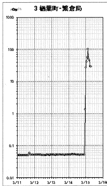
図 C1-4 (1/9) 福島県モニタリングポストの線量率
