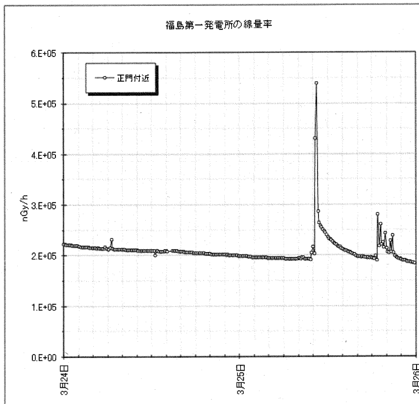
図 C1-1 (7/7) 福島第一発電所構内の線量率 (3月24日—25日)
