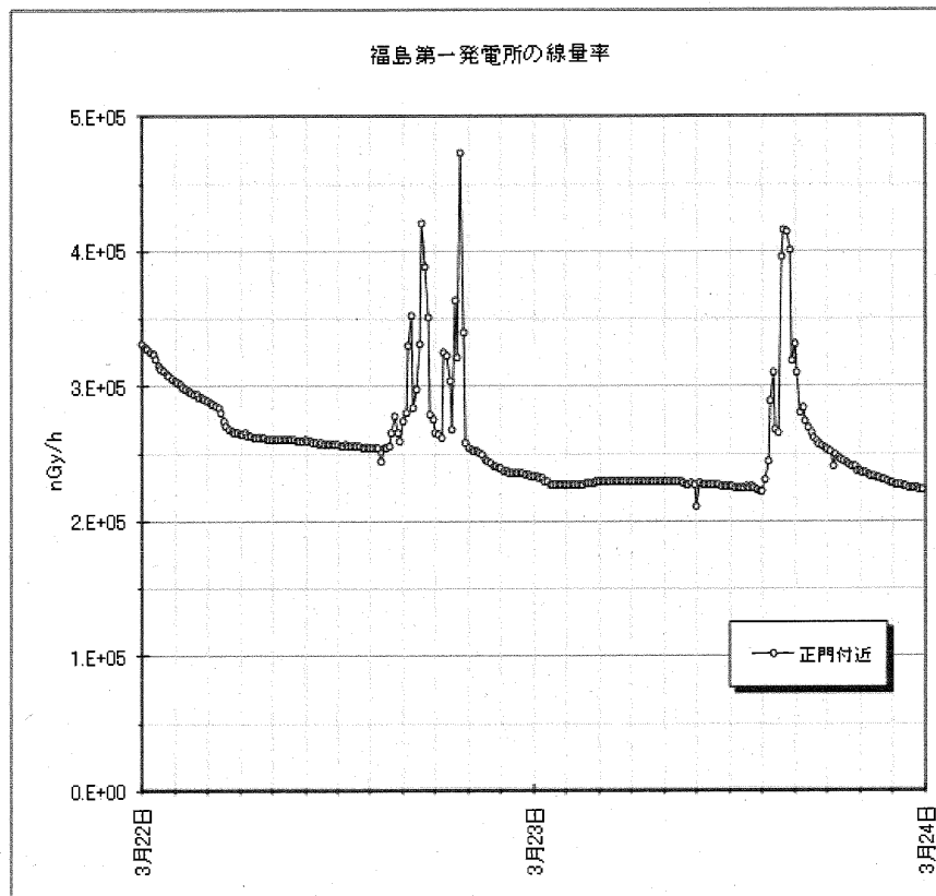
図 C1-1 (6/7) 福島第一発電所構内の線量率 (3月22日—23日)
