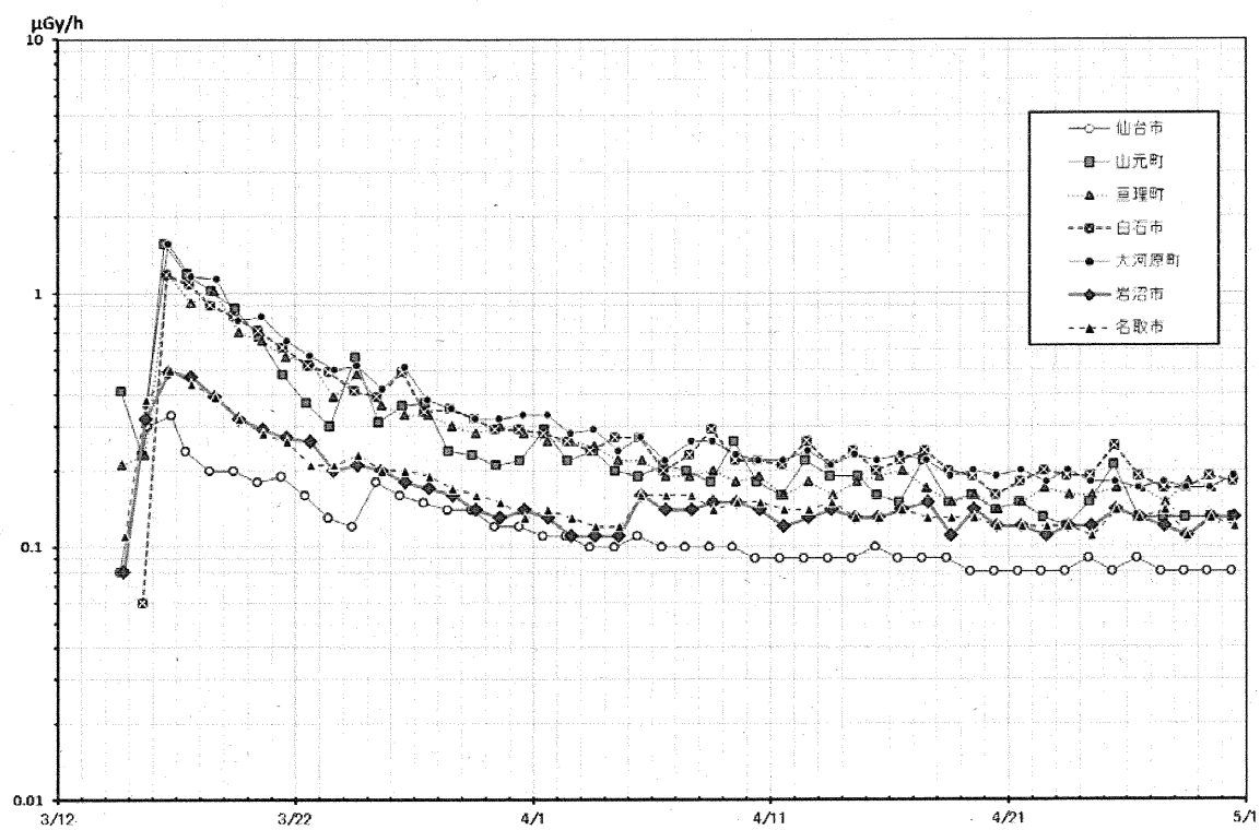
図 C1-9 宮城県各地の線量率 (9)
