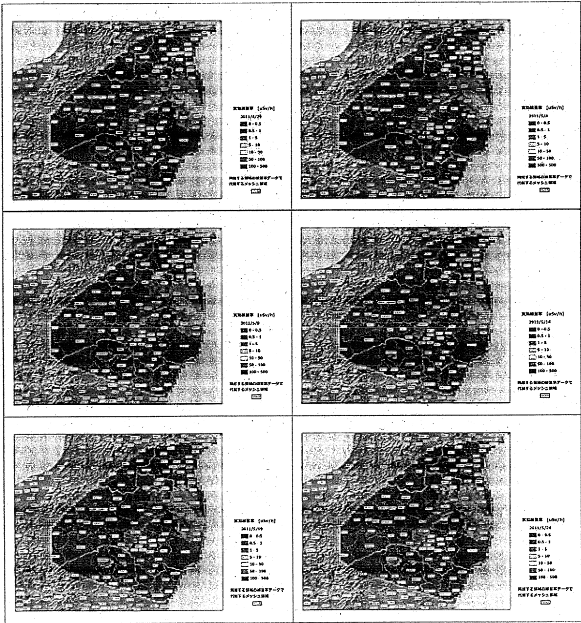
図 8：外部被ばく線量評価に用いる実効線量率マップ (4月29日～5月24日；5日毎).
