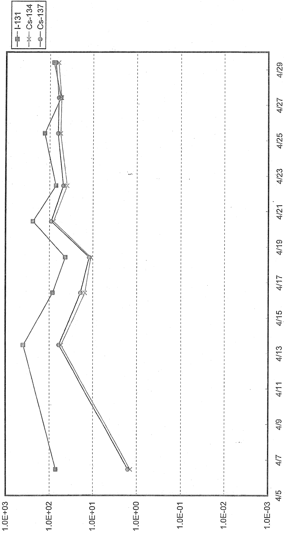
福島第一 1号機サブドレン放射能濃度 (Bq/cm 3 )
